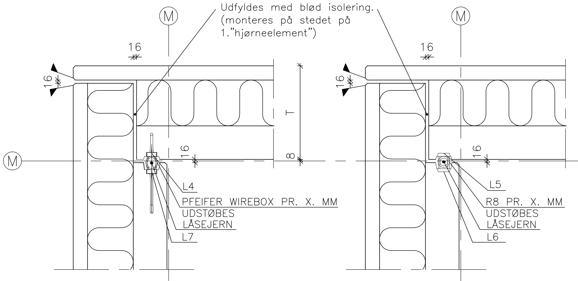
L7/L4 m. PFEIFER WIREBOX
